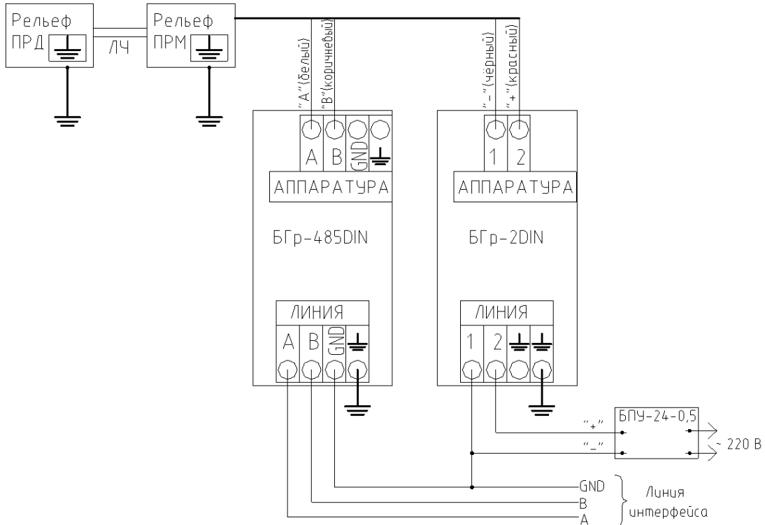
Рисунок 2.11 – Подключение извещателя через блоки грозозащиты «БГр-485DIN» и «БГр2-DIN» для работы в составе сигнализационного комплекса.
